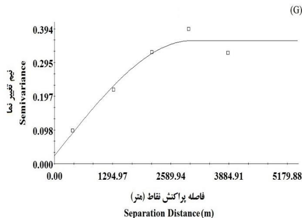
شکل ۲- نیم تغییرنمای همه جهت برای هدایت الکتریکی (مدل نمایی)(الف)، ظرفیت تبادل کاتیونی (مدل نمایی)(ب)، ماده آلی (مدل کرووی) (ج)، اسیدیته (مدل نمایی)(د)، رس (مدل گوسی)(ه)، سیلت (مدل نمایی)(و) و شن خاک (مدل کرووی)(ز).
