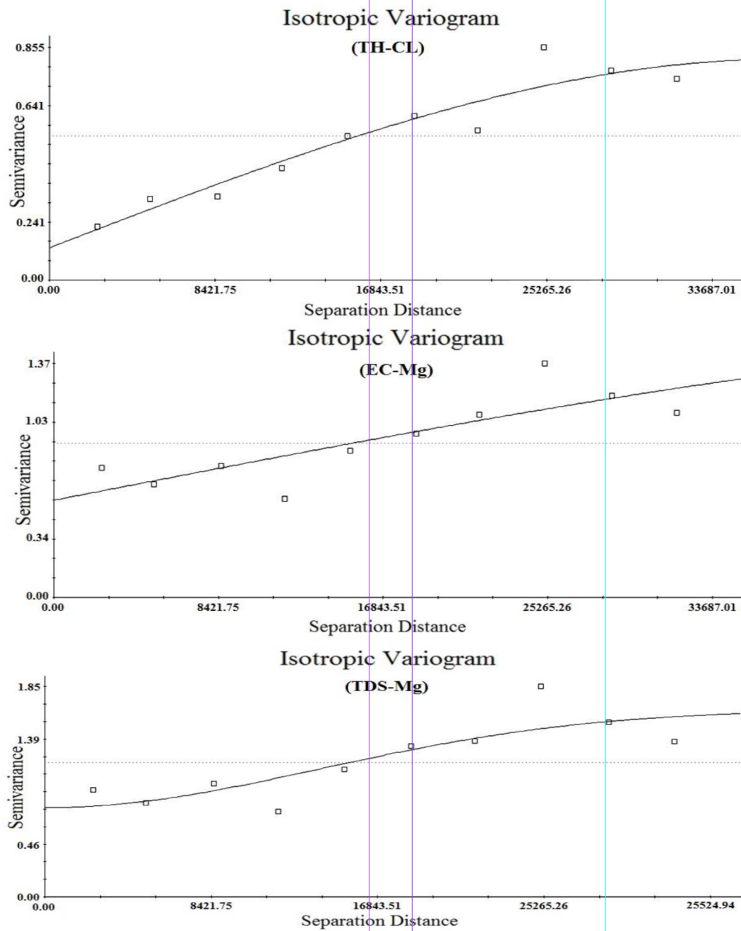
شکل ۳- واریوگرام پارامترهای EC, TH و TDS به همراه پارامترهای کمکی
