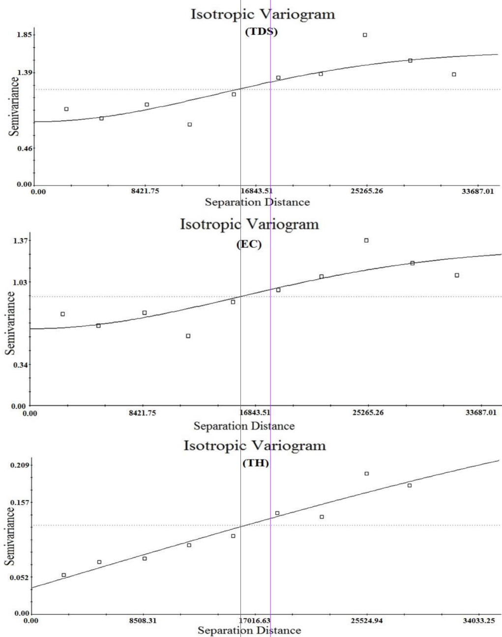
شکل ۲- واریوگرام پارامترهای EC، TH و TDS
