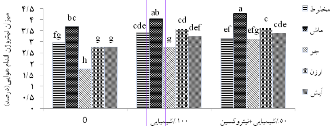
سطوح نیتروژن
