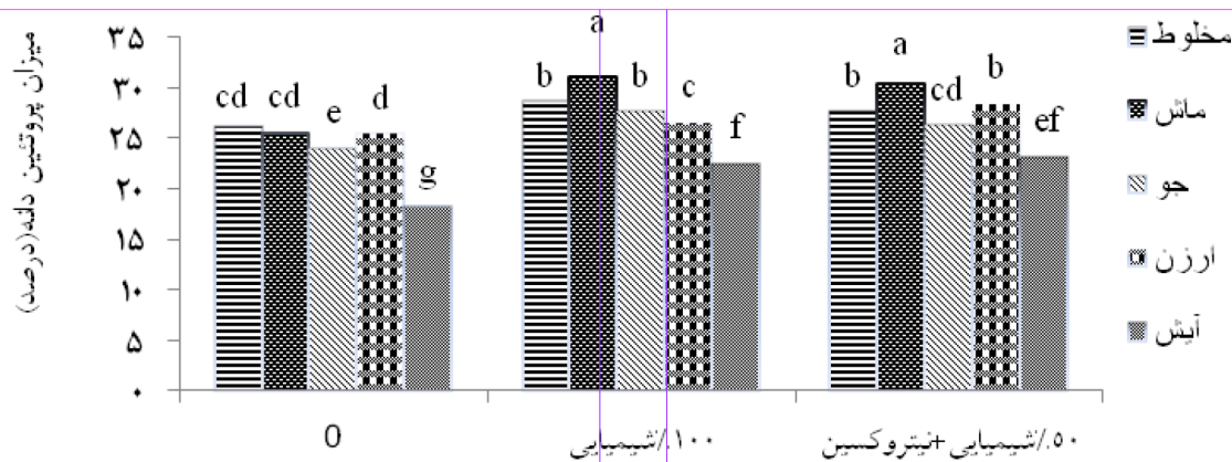
سطوح نیتروژن
