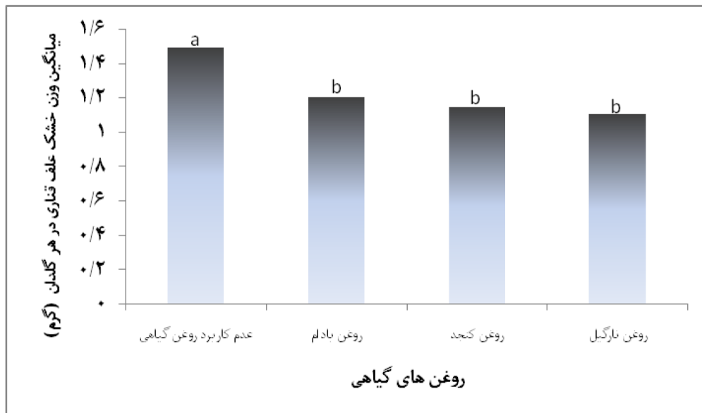
شکل ۲- میانگین وزن خشک علف فناری در هر گلدان (گرم). ستون های با حداقل یک حرف مشترک بر اساس آزمون توکی در سطح ۵ درصد فاقد اختلاف معنی دار هستند. میله های قرار گرفته بر روی هر ستون خطای استاندارد میانگین ها می باشد.
