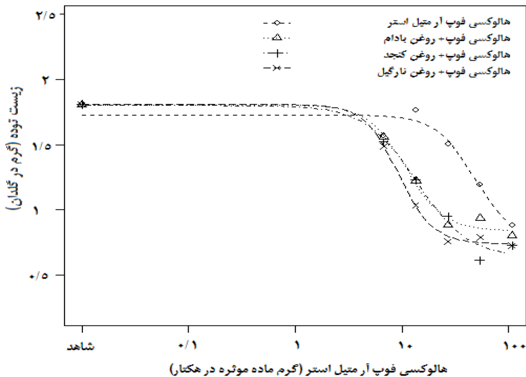
شکل ۳- پاسخ زیست توده علف قناری به مقادیر مختلف علف کش هالوکسی فوپ آرمیتیل استر با و بدون مواد افزودنی. نقاط داده‌های مشاهده شده و خطوط حاصل از برازش معادله سیگموئیدی ۴ پارامتره هستند.
