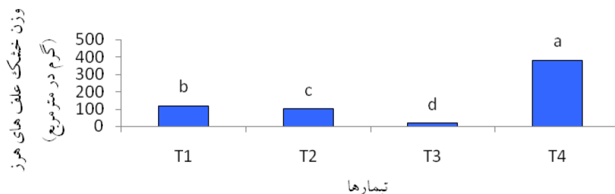
شکل ۵- مقایسه میانگین‌های روش‌های مختلف کنترل علف‌هرز روی وزن خشک علف‌هرز (T 1 ): دوبار وجین‌کن موتوردار، (T 2 ): دوبار وجین‌کن کونویدر، (T 3 ): دوبار وجین‌دستی و (T 4 ): عدم مبارزه.
