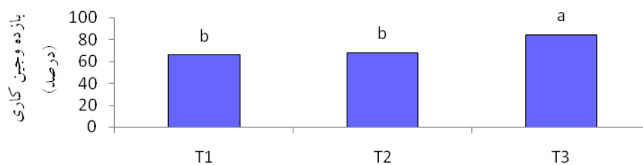
شکل ۳- مقایسه میانگین‌های روش‌های مختلف کنترل علف‌هرز روی راندمان وجین کاری (T 1 ): دوبار وجین‌کن موتوردار، (T 2 ): دوبار وجین‌کن کونویدر، (T 3 ): دوبار وجین‌دستی.
